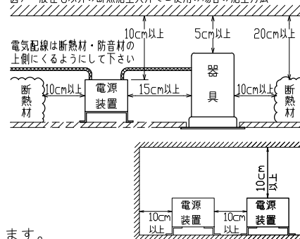
図) 一般住宅以外の断熱施工天井でご使用の場合の施工方法
